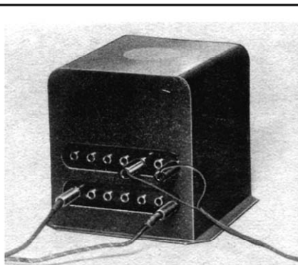
Abb. 4. Das Gehäuse des neuen Vorgelege-Trafos mit versenkten Buchsenreihen
